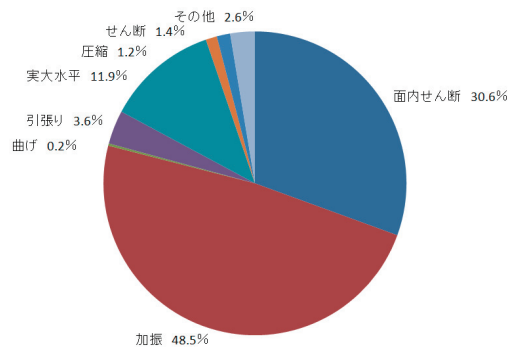
図 19 耐震性能に関する実験の内容構成（日本建築学会）
